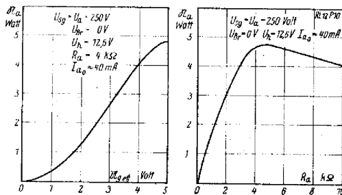
NF-Wechselstromleistung als Funktion der Gitterwechselspannung und als Funktion von R_a bei Aussteuerung bis zum Gitterstrom-Einsatz
