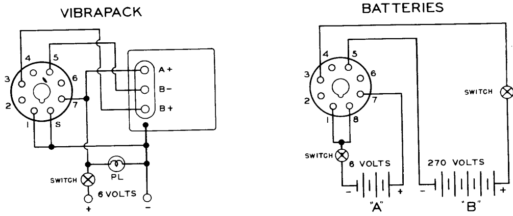
Fig. 2. Wiring diagrams DC power plug.
